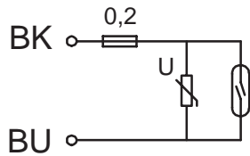
Anschlußbild
